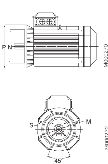
Типоразмеры 225-400
