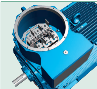
Рис. 10. Кабельные зажимы для двигателей типоразмеров 355-400
