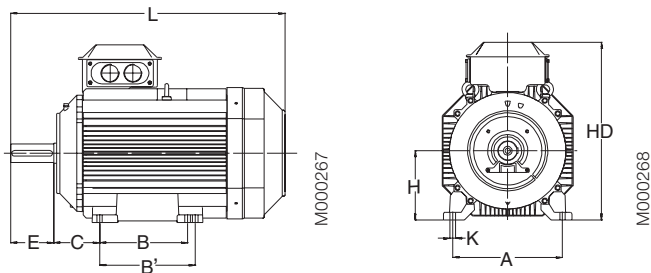
Типоразмеры 90-200
