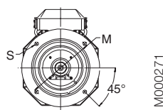
Типоразмеры 90-200
