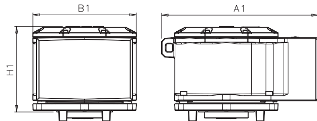
Двигатели типоразмеров 355-400
