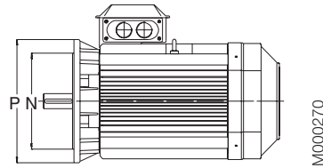
Типоразмеры 225-250
