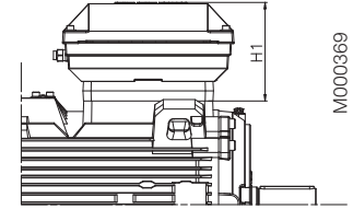
Двигатели типоразмеров 200 - 250
