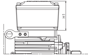
Двигатели типоразмеров 80-132
