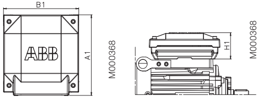
Двигатели типоразмеров 80 - 132
