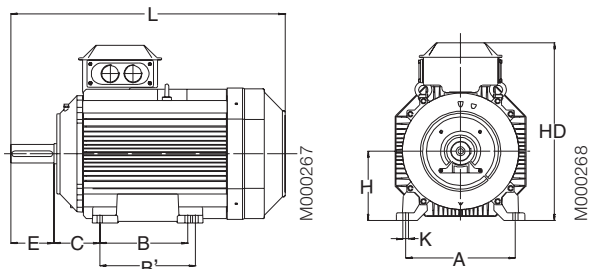
Двигатель с монтажом на лапах IM 1001, IM B3
