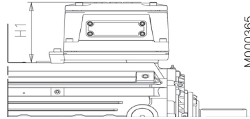
Двигатели типоразмеров 160 - 180
