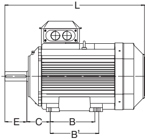
Удлинение вала
