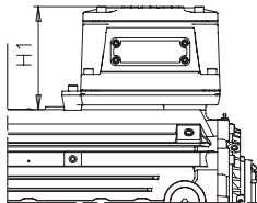
Двигатели типоразмеров 280-315
